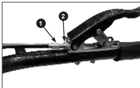
Рис. 44. Регулировка троса включения хода 1. Винт регулировочный 2. Контргайка
