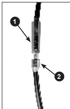
Рис. 43. Регулировка троса включения хода 1. Контргайка 2. Винт регулировочный
