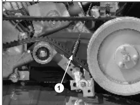
Рис. 42. Пружина троса включения хода 1. Пружина троса включения хода
