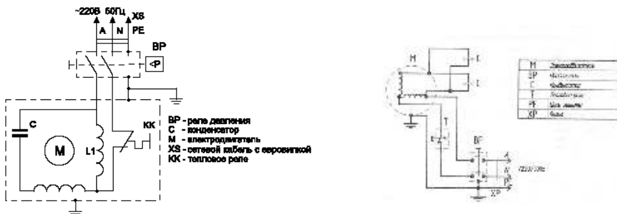
Рис. 2. Схема электрическая принципиальная
