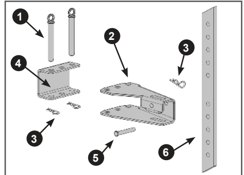
Рис. 19. Установка сошника
