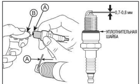
Рис. 38. Проверка межэлектродного зазора А - зазор В - щуп
